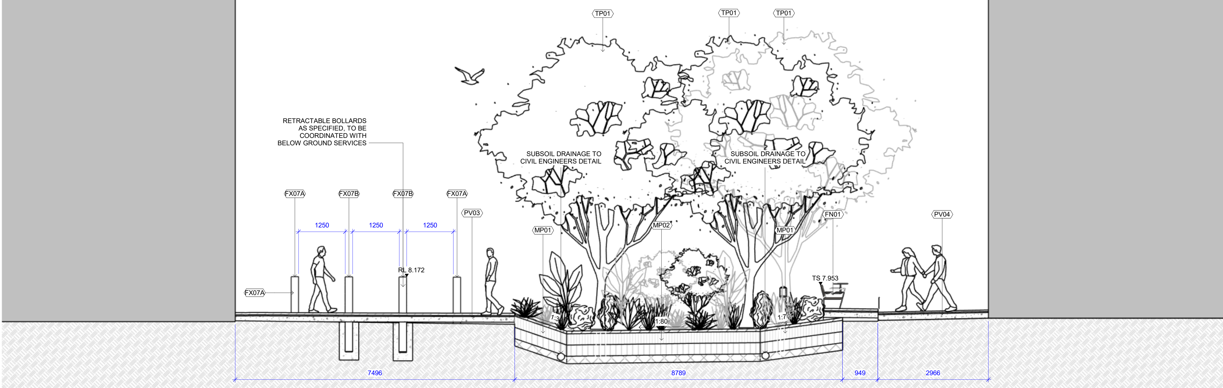
1 WSUD RAINGARDEN SECTION 1 1 : 50
