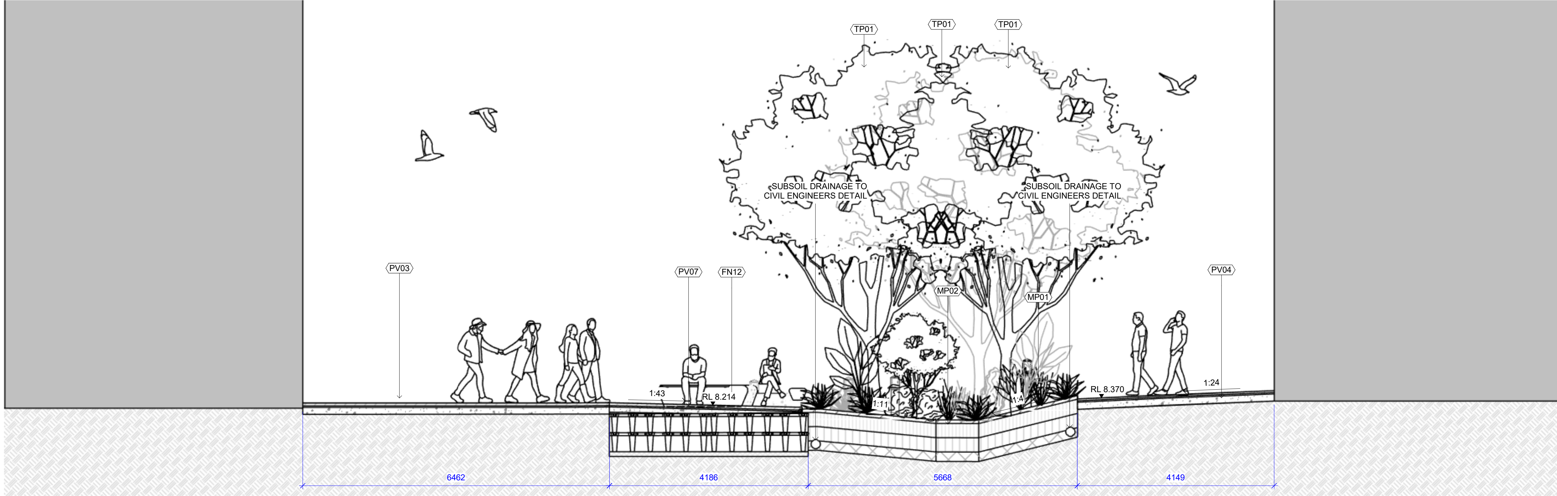
2 WSUD RAINGARDEN SECTION 2 1 : 50
